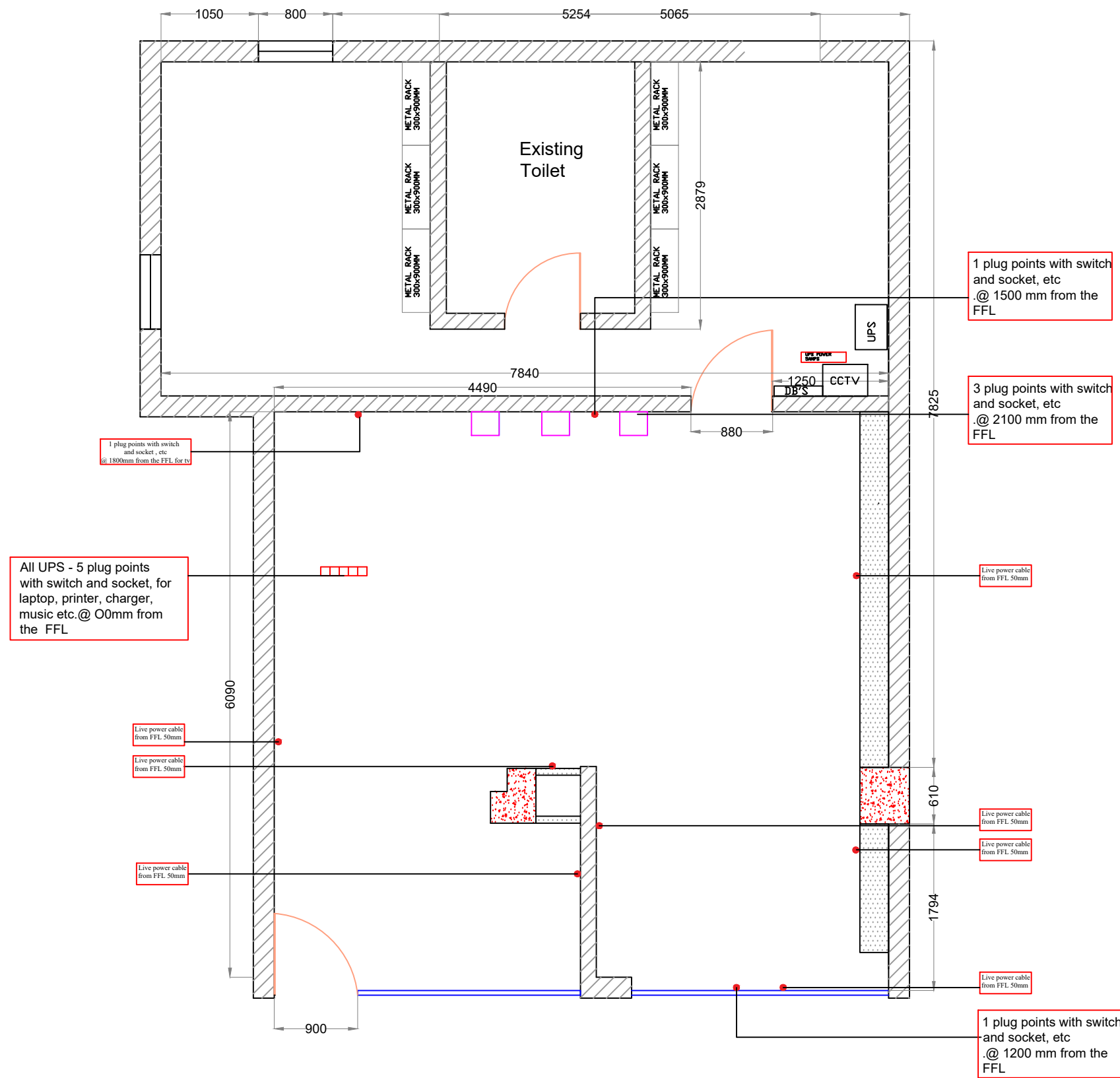
POWER LAYOUT A-1.1 SCALE: NTS
