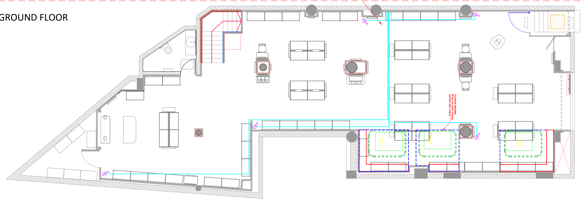
CCTV LAYOUT Scale: 1 : 75
